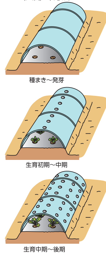
図3 トンネルの換気(穴開け)方法
